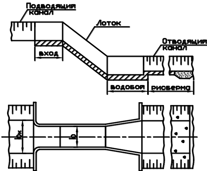
Рисунок 4.1 – Схема быстротока
