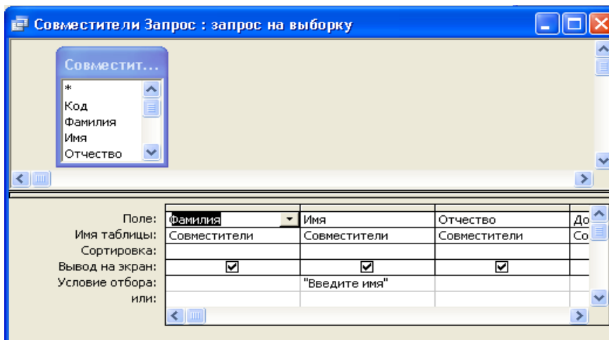
Рисунок 8 Экран Конструктора запросов
