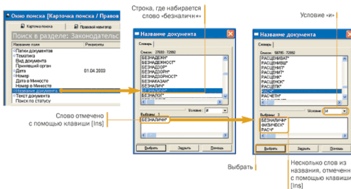
Рис.2.8. Поиск документа по общим словам
