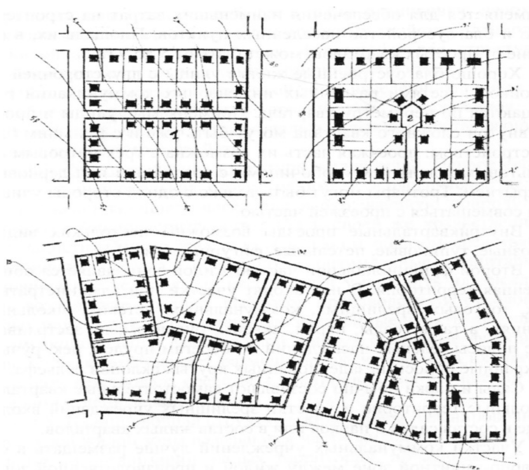
Рисунок 13 – Сложные квартиры участковой застройки: 1 – со сквозным проездом; 2 – с тупиковым проездом; 3 – с петельным проездом; 4 – с фигурным проездом
