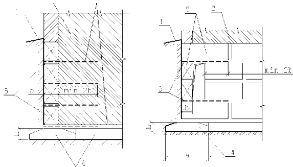
Рисунок 2.5 – Примыкание кирпичной стены к стене из бетонных блоков (а) и устройство вводов (б)
