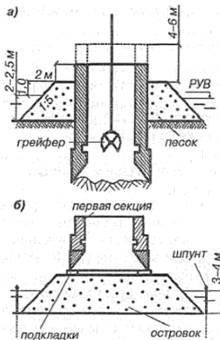
Рисунок 2.45 – Устройство островка: а – без ограждения; б – в ограждении
