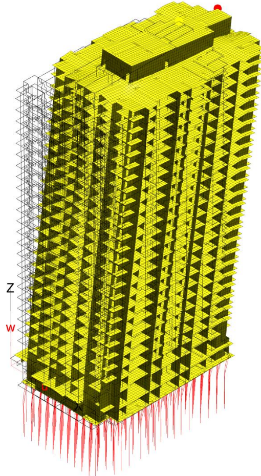
Рисунок 1.7 – Деформации здания по 2-й форме собственных колебаний
