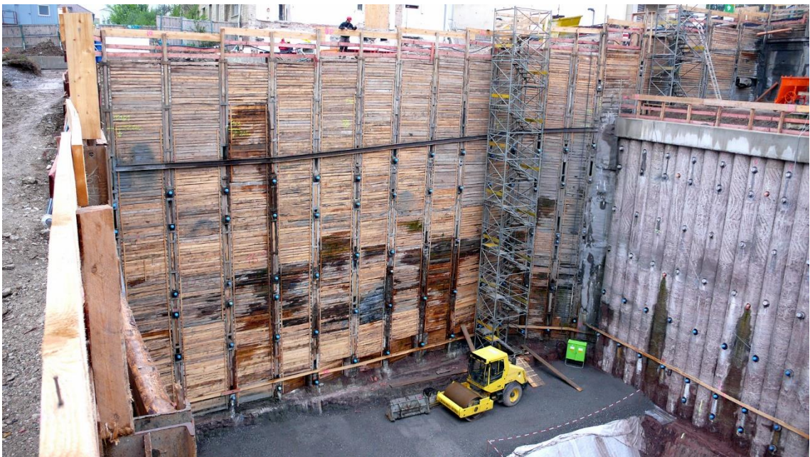
Рисунок 6.4 – Госпиталь Св.Ольги (Штутгарт, Германия) Сочетание различных типов ограждения котлована и высачивание грунтовых вод по трещинам в породах
