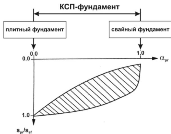
Рисунок 2.27 – Изменение свайно-плитного коэффициента и область использования расчетных моделей
