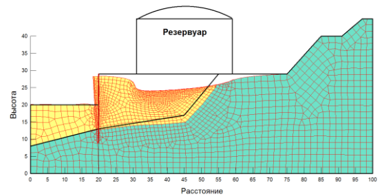
Рисунок 2.69 – Расчет деформаций по плоским (2D) моделям
