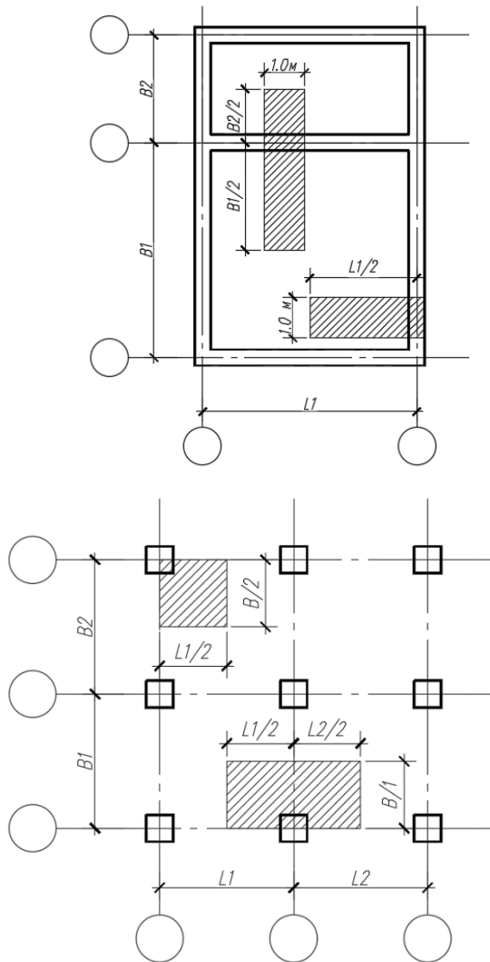
Рисунок 1.1 – Схема расчета грузовых площадей
