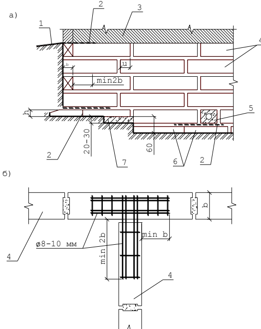
Рисунок 2.4 – Перевязка наружных и внутренних стен а – блоком; б --арматурными сетками:
