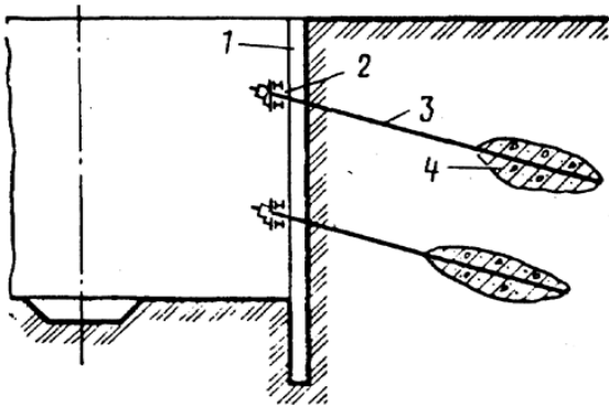
Рисунок 2.40 – Анкерное крепление котлована: 1 – свая крепления котлована; 2 – пояс из двух двутавров; 3 – тяга анкера; 4 – заделка анкера
