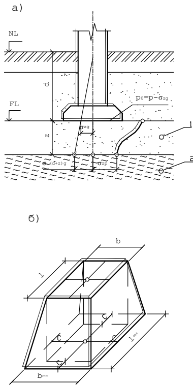
Рисунок 2.9 - К проверке прочности слабого подстилающего слоя
