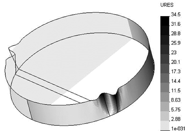
Рисунок 1.12 – Расчетные деформации стенок РВС
