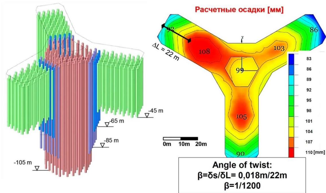
Рисунок 2.62 – Схема распределения свай разной длины в пределах фундамента «Кингдом Тауэр» с указанием изополей расчетных осадок фундаментной плиты
