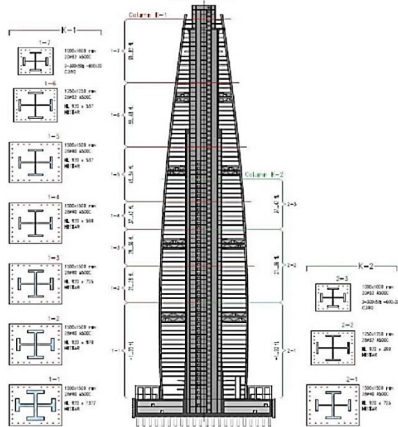
Рисунок 2.51 – Схема изменения поперечного сечения несущих колонн здания «Лакhta Центр» с ростом этажности
