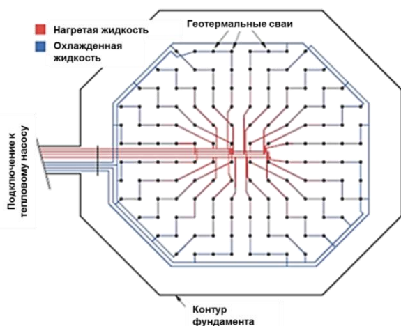
Рисунок 2.31 – Схема свайного поля с применением геотермального контура в сваях
