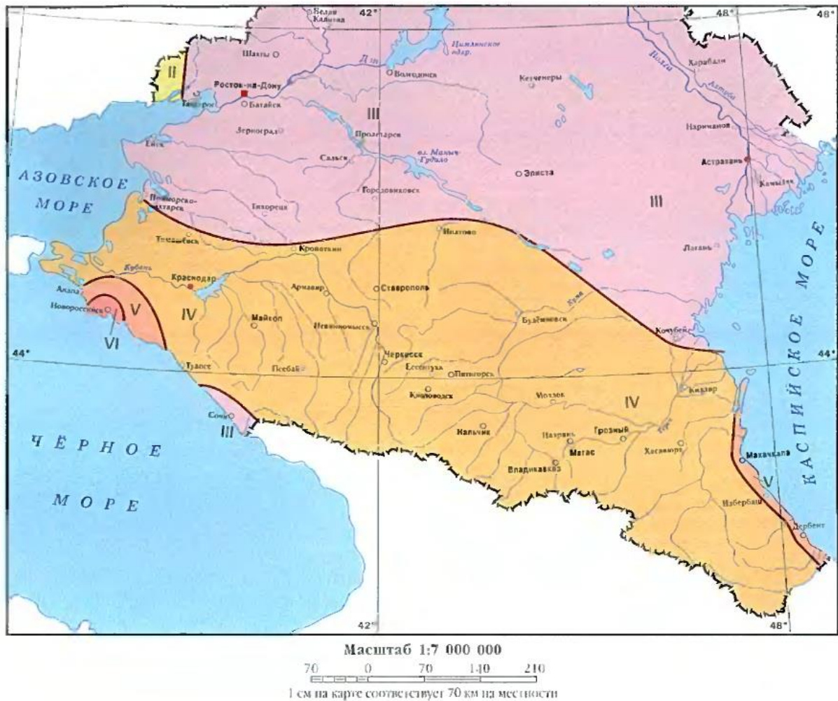
Рисунок 1.5 – Районирование территории Кавказа по давлению ветра
