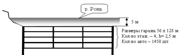
Рисунок 2.36 – Схема устройства четырёхуровневого гаража под рекой по методу «стена в грунте»
