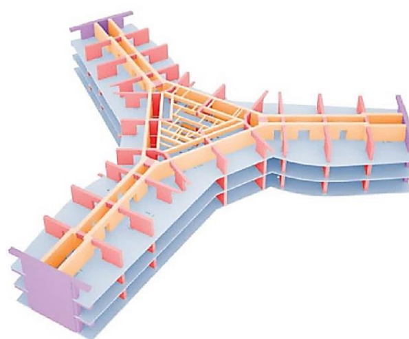
Рисунок 2.61 – Схема расположения основных несущих элементов высотного здания «Кингдом Тауэр»
