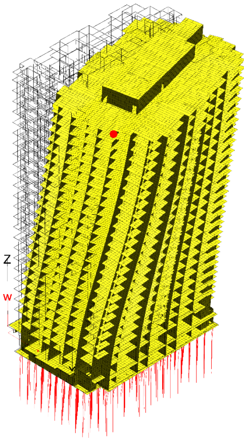
Рисунок 1.6 – Деформации здания по 1-й форме собственных колебаний
