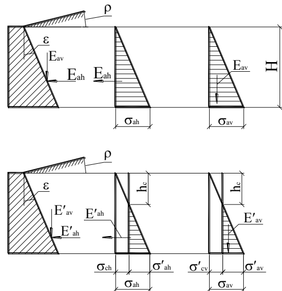
Рисунок 4.1 - К определению активного давления грунта на стенку а – несвязного; б – связного
