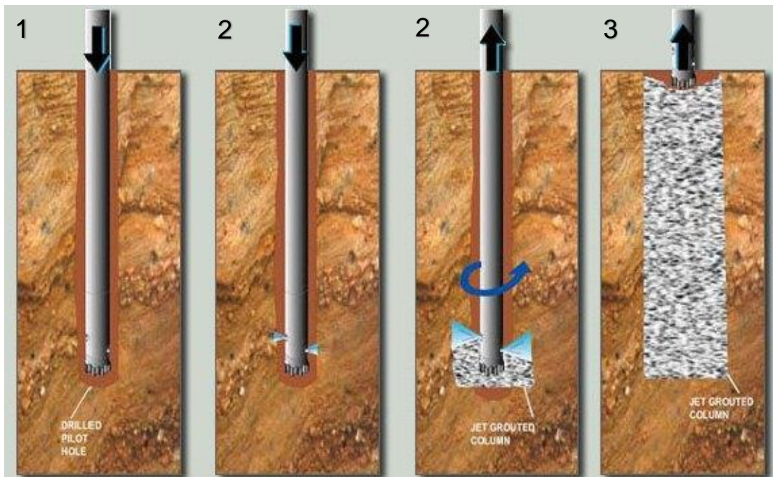
Рисунок 2.18 - Цементация грунтов
