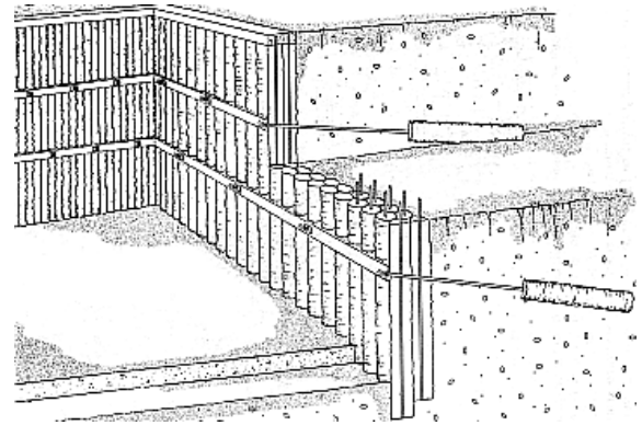
Рисунок 2.41 – Анкерное крепление котлована
