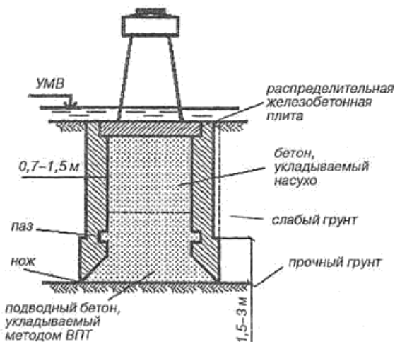
Рисунок 2.43 – Общий вид опускного колодца
