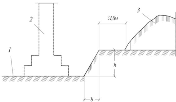
Рисунок 6.1. - Котлован с естественными откосами: 1 – дно котлована; 2 – очертания будущего фундамента; 3 – вынутый грунт
