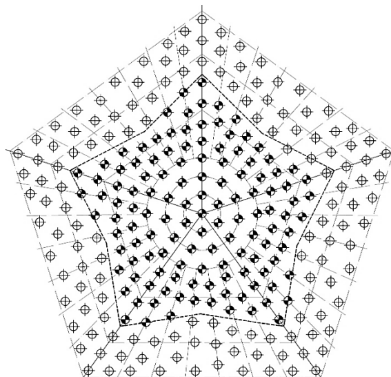
Рисунок 2.56 – Схема расположения свай в составе фундамента здания «Лахта Центр»
