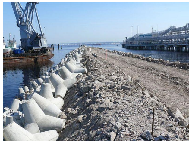
Рисунок 1.10 – Крепление берега тетраподами
