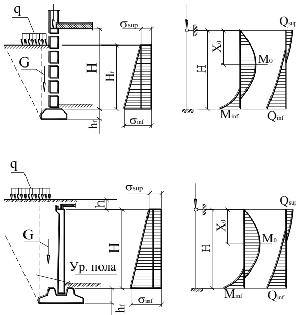
Рисунок 4.3: К определению расчетных усилий в стенах подвалов
