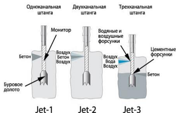
Рисунок 5.2 – Создание грунтоцемента с помощью систем Jet-1, Jet-2 и Jet-3
