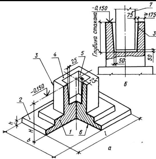
Рисунок 2.2: Монолитный железобетонный столбчатый фундамент: а – общий вид; б – подколонник; 1 – плитная часть (одно-, двух- или трёхступенчатая) 2 – подошвенная плита; 3 – подколонник стаканного типа; 4 – обрызг фундамента; 5 – стакан; 6 – подошва фундамента; 7 – колонна.
