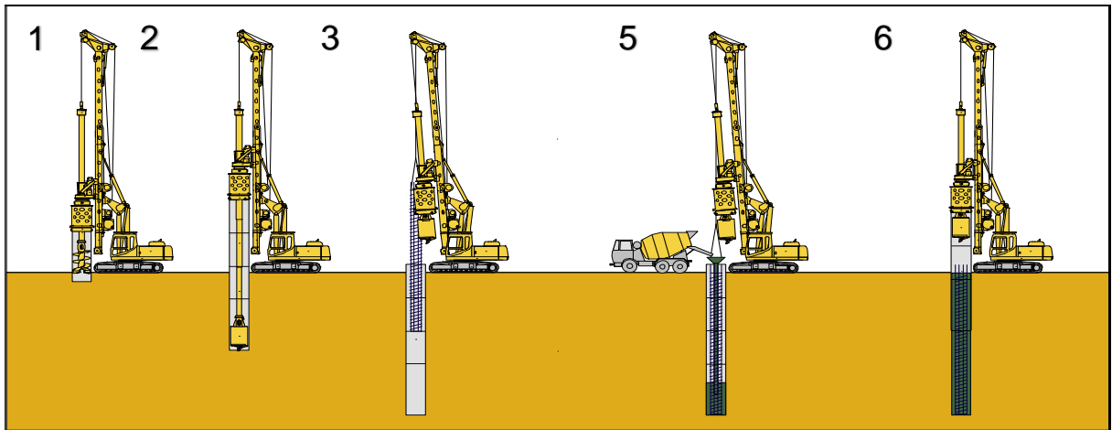
Рисунок 2.16 - Бурунабивные сваи под обсадной трубой с келли-штангой
