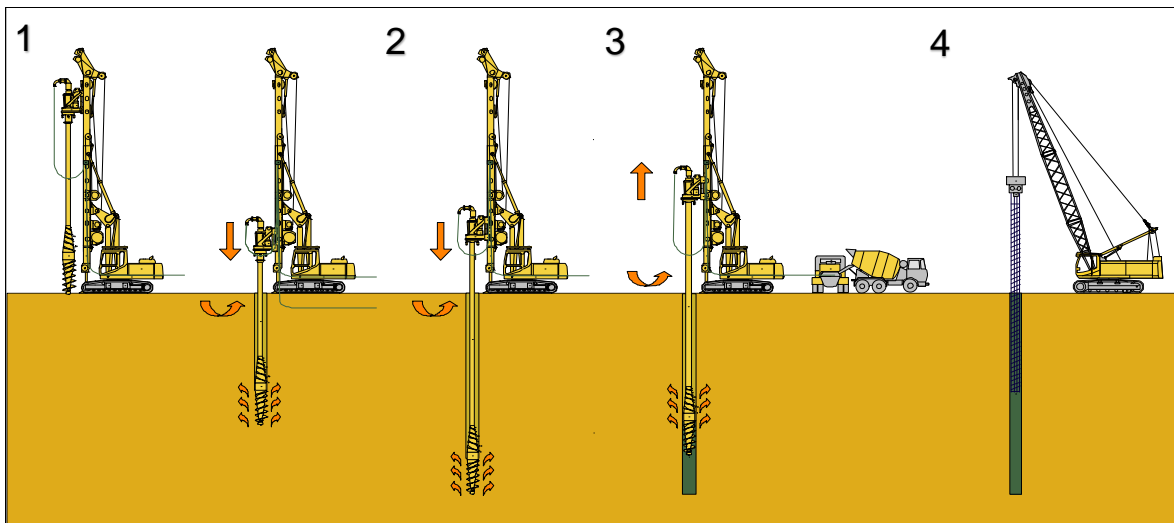
Рисунок 2.14 - Технология DDS
