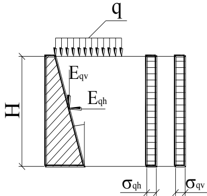
Рисунок 4.2 - К определению давления грунта от нагрузки на поверхности засыпки
