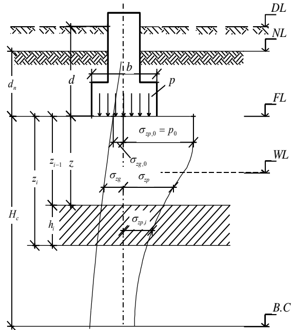
Рисунок 2.10 - Схема распределения вертикальных напряжений в линейно-деформируемом полупространстве:
