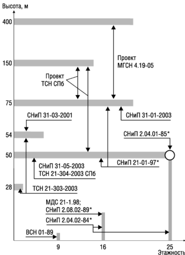
Рисунок 2.21 – Ограничительные области в нормативных документах РФ по высотности и этажности зданий и сооружений
