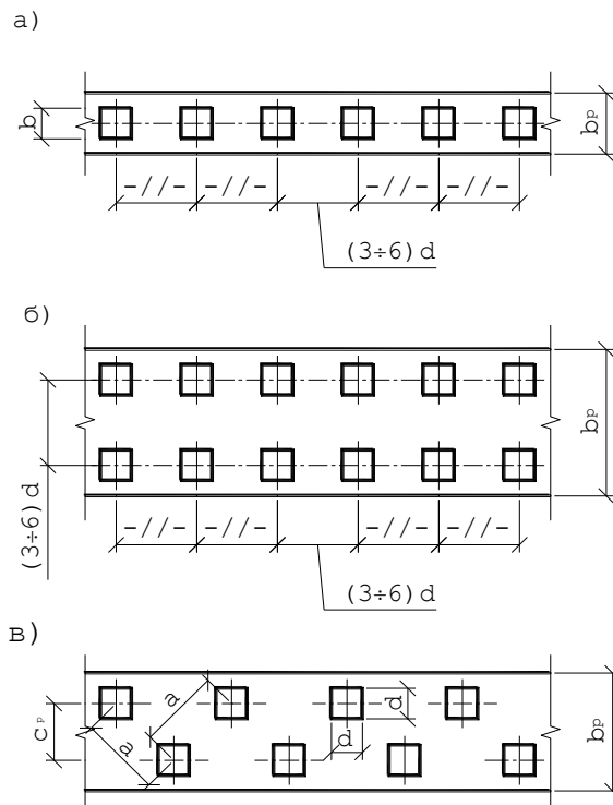
Рисунок 2.12 - Расположение свай в плане под стенами
