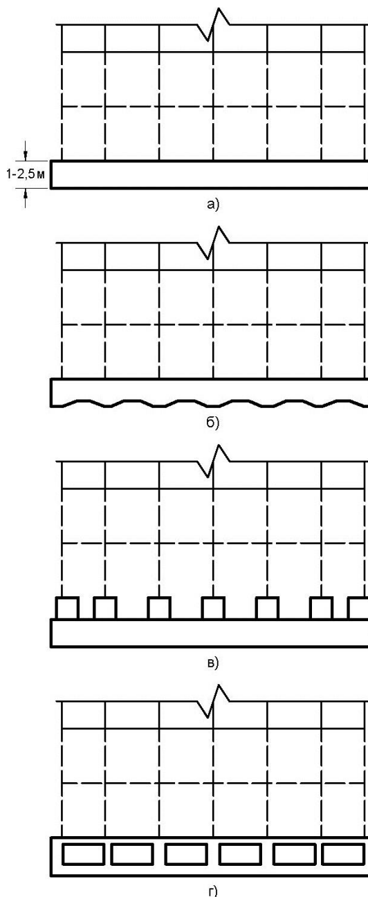
Рисунок 2.23 – Конструкции сплошной монолитной железобетонной плиты:
