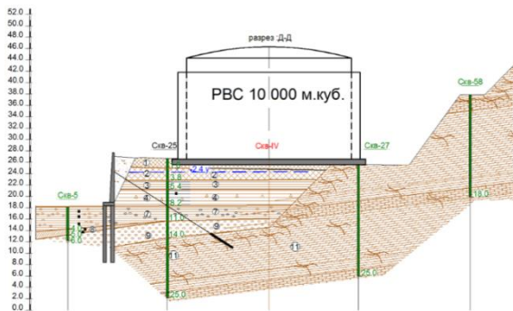
Рисунок 2.66 – Резервуар для нефтепродуктов (РН Туапсинский НПЗ)
