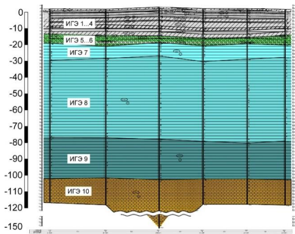
Рисунок 2.54 – Инженерно-геологические условия площадки строительства здания «Лахта Центр»: ИГЭ 1 – 4 – комплекс морских и озерных отложений; комплекс озерно-ледниковых отложений; ИГЭ 5,6 – ледниковые отложения; ИГЭ 7 – 10 – верхнепротерозойские котлинские отложения
