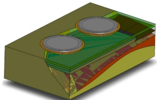
Рисунок 2.68 – Пространственная (3D) модель основания резервуаров
