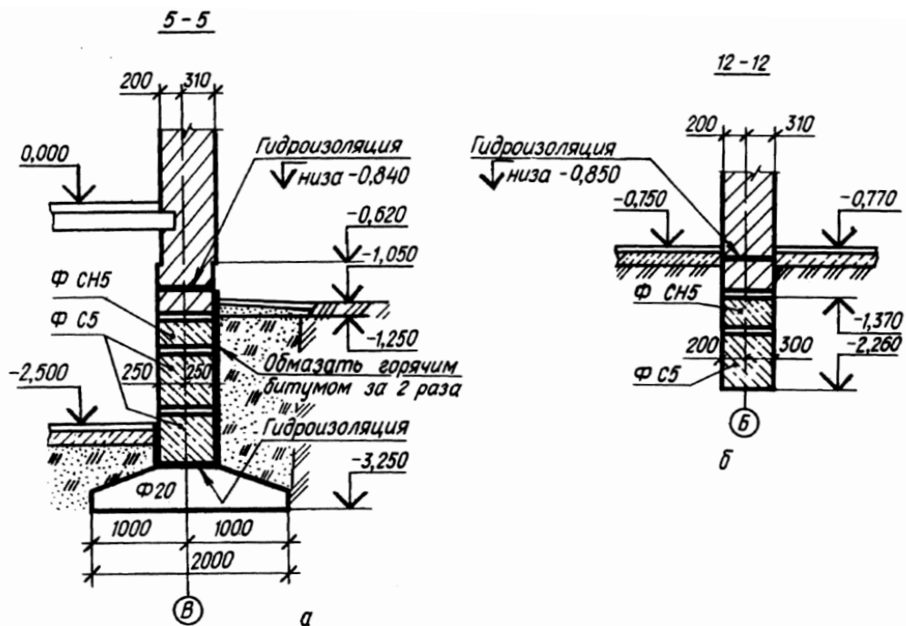
Рисунок 10.5 - Образец выполнения чертежа поперечных сечений фундаментов:
