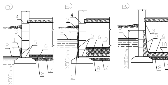
Рисунок 7.2 - Гидроизоляция подвальных помещений при небольших (а) и при больших (б,в) напорах подземных вод;
