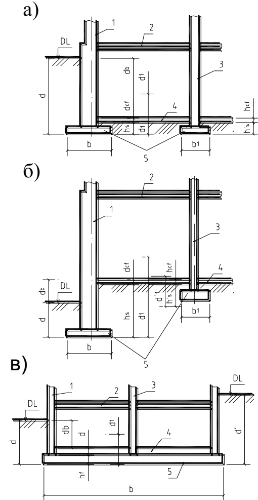
Рисунок 2.7 - К определению глубины заложения фундаментов
