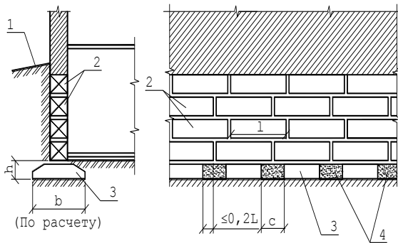
Рисунок 2.8 - Прерывистый фундамент: 1 – поверхность грунта; 2 – бетонные блоки; 3 – фундаментные плиты; 4 – промежутки между плитами, заполненные грунтом
