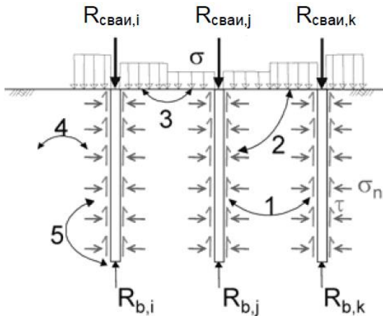
Рисунок 2.26 – Взаимодействия между КСПФ и грунтами основания:
