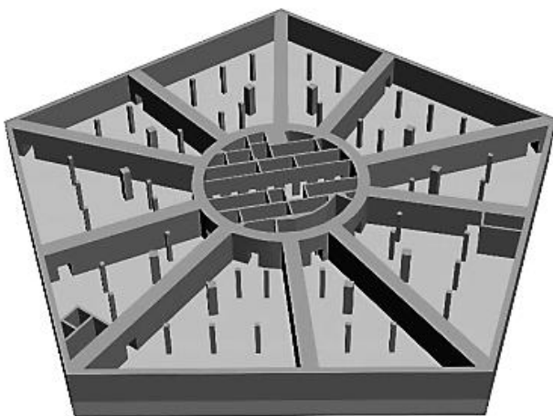
Рисунок 2.55 – Пространственная схема коробчатого фундамента здания «Лахта Центр»
