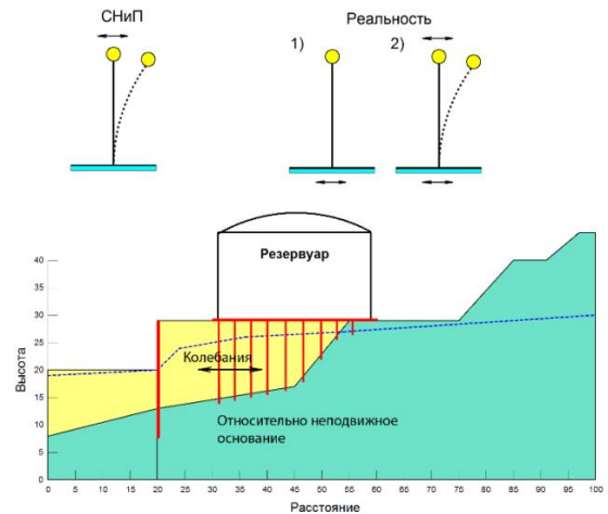
Рисунок 2.67 – Сравнение расчетной модели СНиП и реальности
