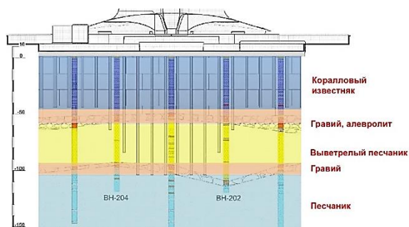
Рисунок 2.59 – Грунтовые условия площадки строительства «Кингдом Тауэр»
