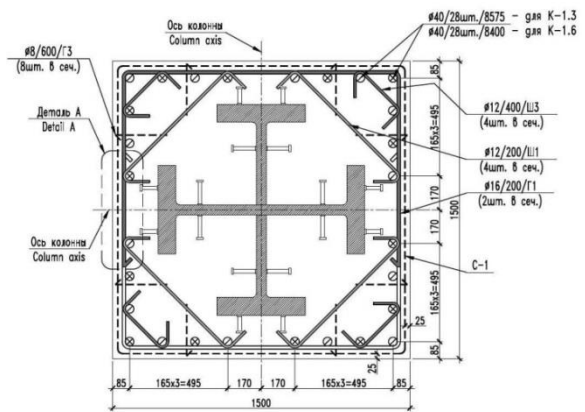
Рисунок 2.52 – Типовое поперечное сечение колонны
