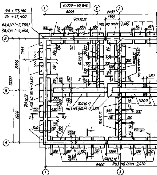
Рисунок 10.2 – Условные обозначения на плане фундаментов
