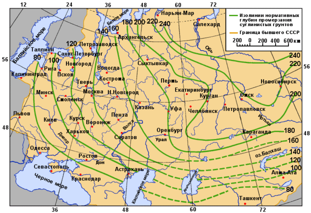
Рисунок 2.6 – Схематическая карта нормативных глубин промерзания (изолинии нормативных глубин промерзания, обозначенные пунктиром, даны для малоисследованных районов)
