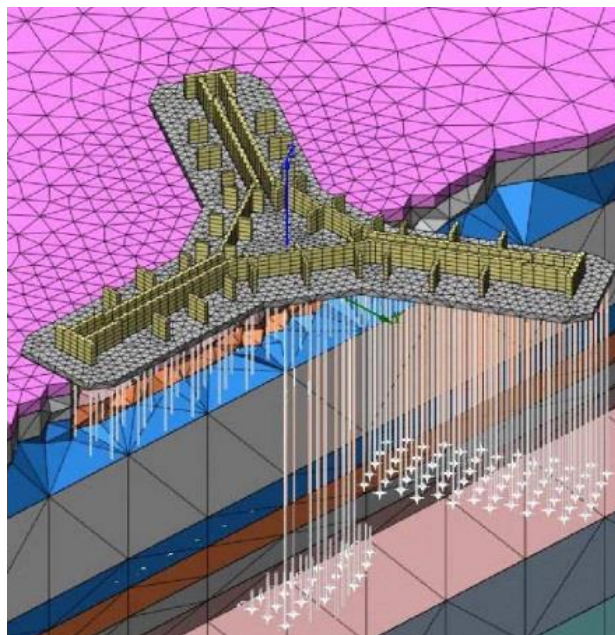
Рисунок 2.60 – Фрагмент расчетной модели высотного здания с выделением основных несущих элементов в уровне заделки свай переменной длины в фундаментную плиту
