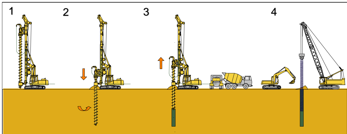
Рисунок 2.13 - Технология CFA
