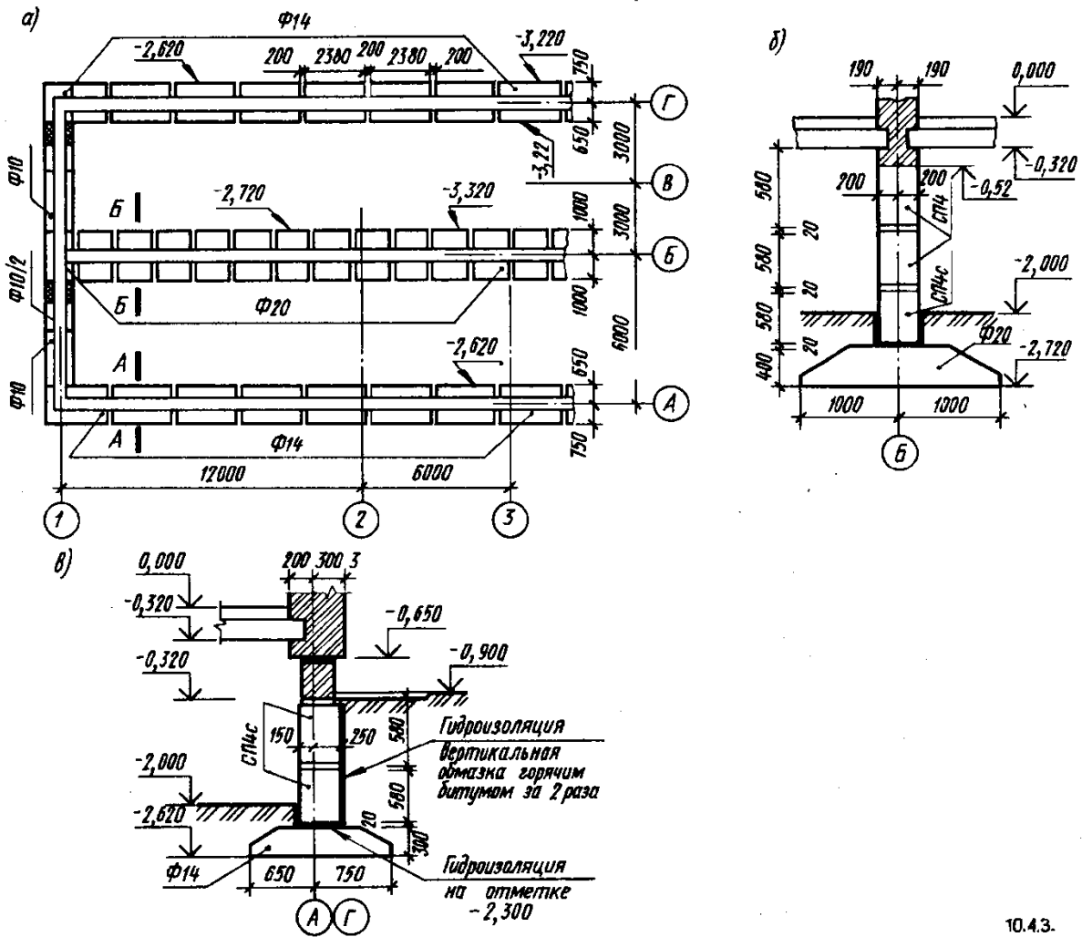
Рисунок 10.8 - Образец выполнения чертежей сборных фундаментов
