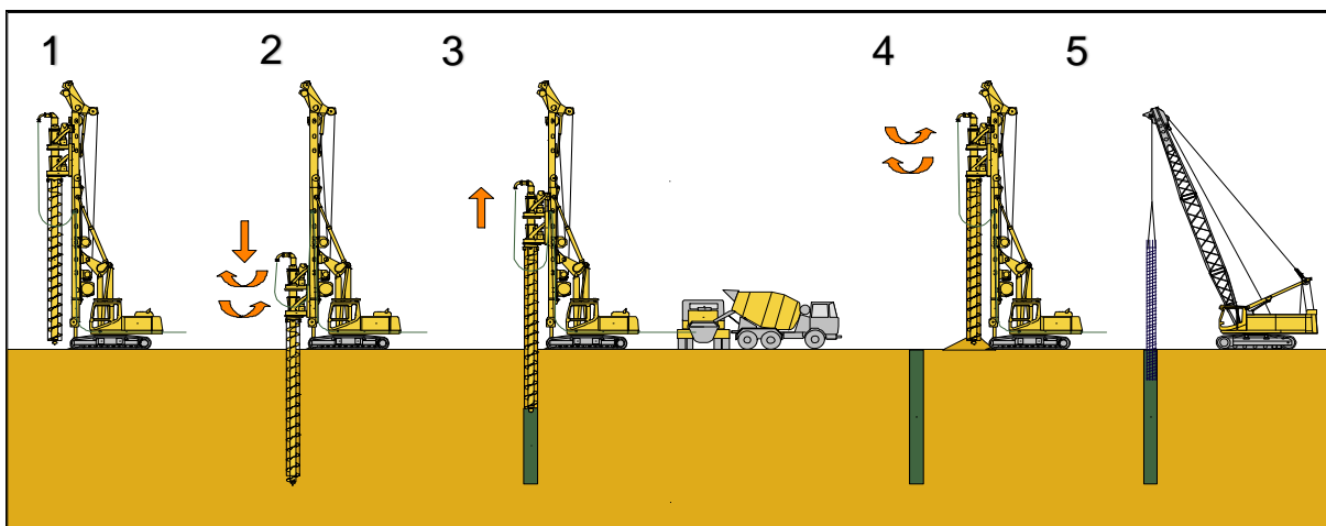
Рисунок 2.15 - Технология CFA
