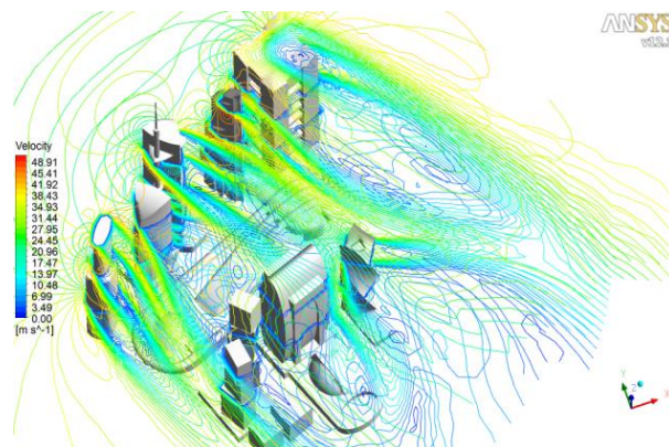
Рисунок 1.9 – Обтекание воздухом высотного объекта прямоугольной формы
