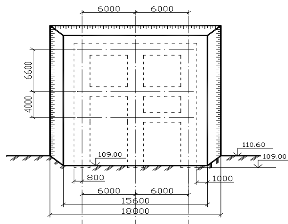
Рисунок 6.2 – План котлована, совмещенный с разрезом
