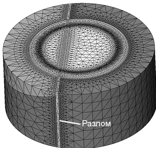
Рисунок 1.11 – Расчетная модель МКЭ системы «основание-фундамент-резервуар»
