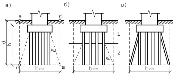
Рисунок 2.20 - Схемы условных фундаментов для расчета по второй группе предельных состояний
