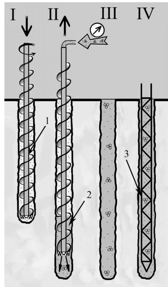
Рисунок 2.19 - Технологическая схема устройства свай «micro CFA»:
