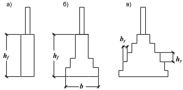
Рисунок 2.1 – Конструкции жестких фундаментов: а – минимальной ширины; б – обычной; в – уширенной
