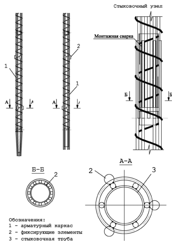
Рисунок 5.1 - Армирование буронагреционной сваи
