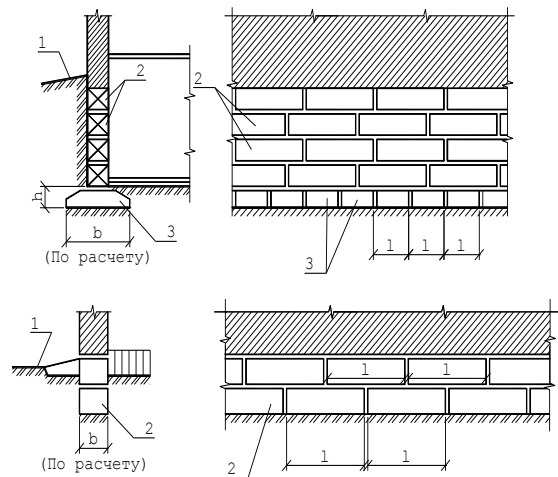
Рисунок 2.3 – Сборный ленточный фундамент а – для здания с подвалом; б – для здания без подвала
