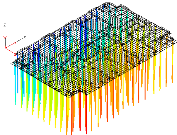
Рисунок 1.8 – Пример эпюры усилий в сваях
