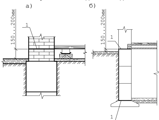
Рисунок 7.1 - Изоляция сырости стен бесподвального здания (а) и стен подвального помещения (б);
