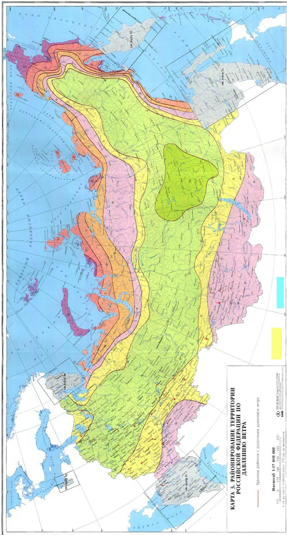
Рисунок 1.4 – Районирование территории России по давлению ветра
