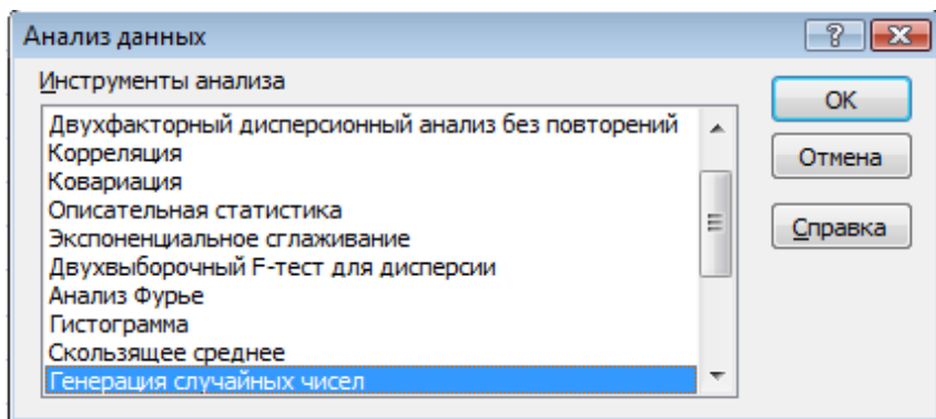
Рисунок 1 – Анализ данных
