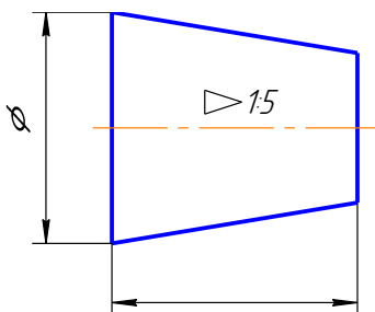
Рисунок 3.32 – Пример указания размеров при двух диаметрах
