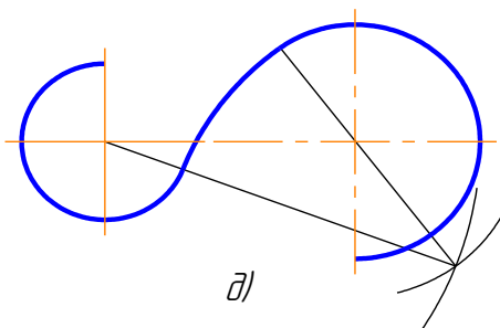
Рисунок 3.15 – Построение сопряжения при смещенном сопряжении
