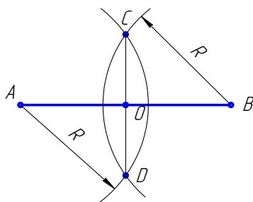
Рисунок 3.2 – Построение перпендикуляра к середине отрезка
