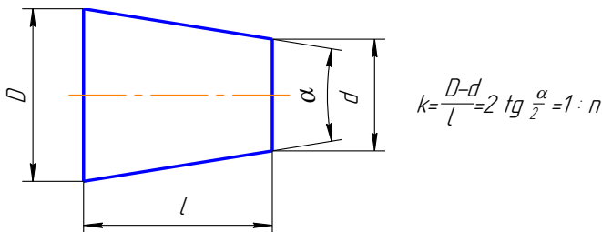
Рисунок 3.29 – Построение конусности
