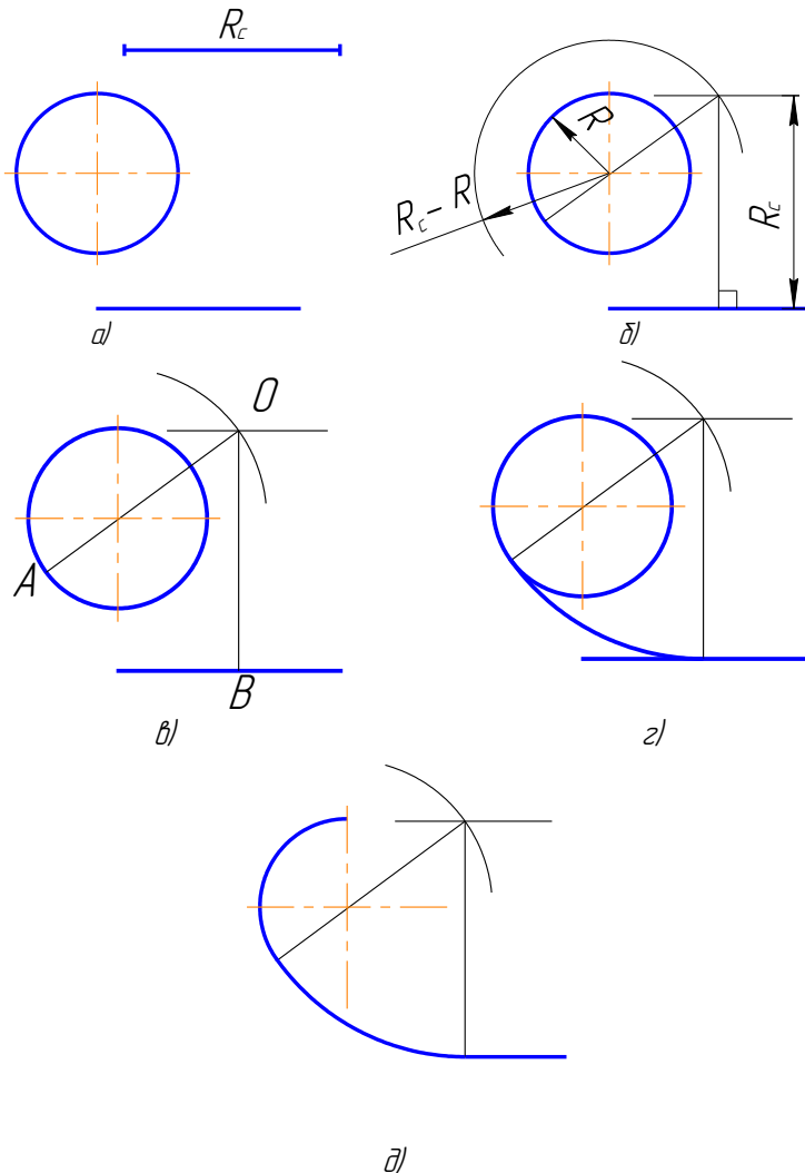
Рисунок 3.11 – Построение сопряжения между дугой окружности и прямой линии в случае, когда заданная окружность
