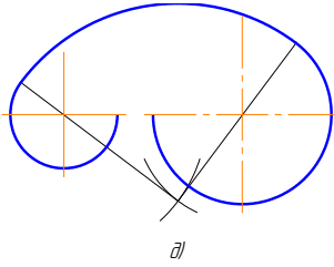
Рисунок 3.14 – Построение заданной окружности находящейся внутри сопрягающей дуги (внутреннее сопряжение)
