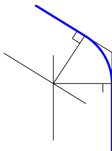
Рисунок 3.9 – Пример 3 построения сопряжения
