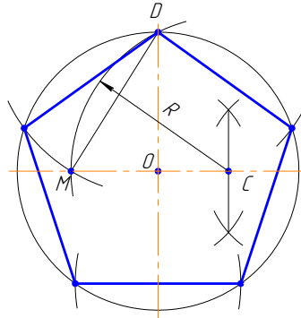
Рисунок 3.4 – Деление окружности на пять равных частей
