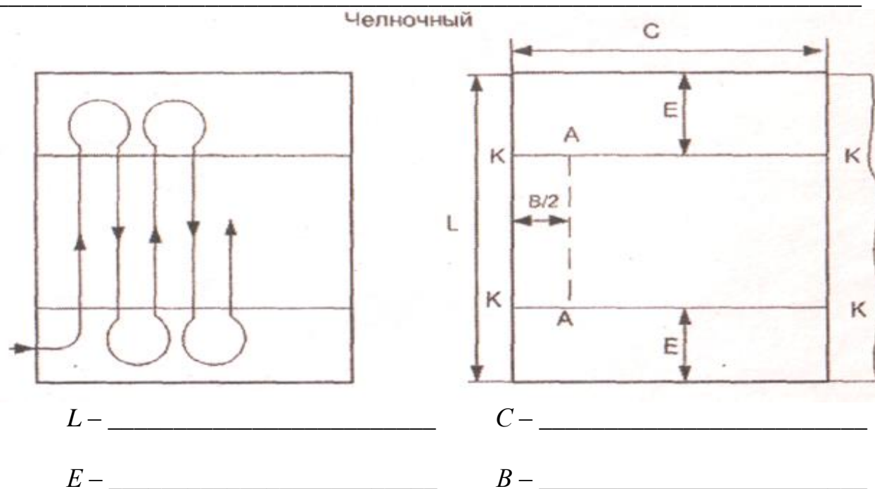
Рисунок 1 – Схема движения и подготовки поля к культивации при способе движения агрегата челночный
