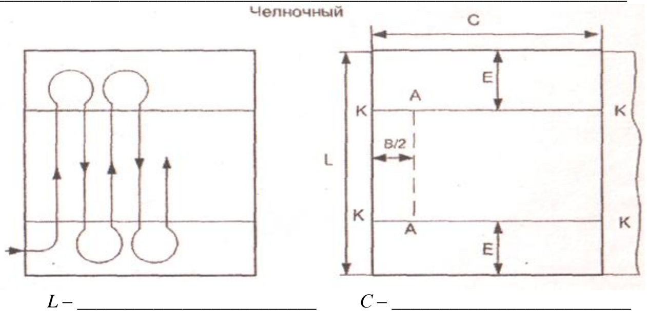
Рисунок 1 – Схема движения и подготовки поля к опрыскиванию при способе движения агрегата челночный
